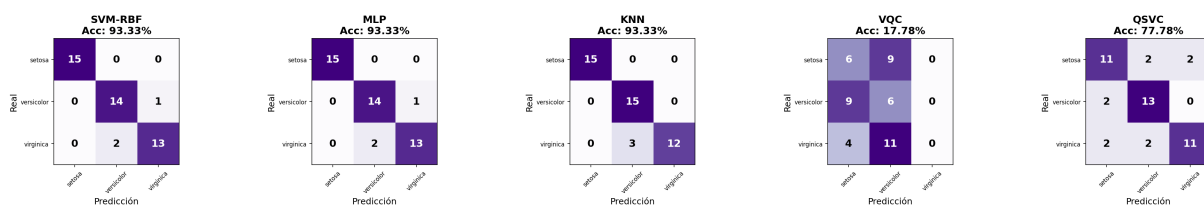
Figura 5: Matrices de confusión para los cinco modelos evaluados sobre el conjunto de test de Iris.
