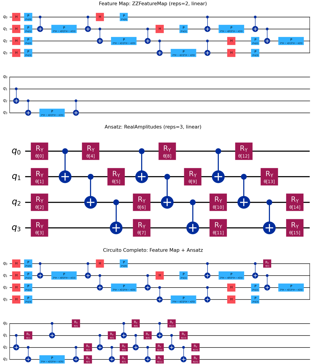
Figura 1: Circuitos cuánticos utilizados. Arriba: ZZFeatureMap (reps=2). Centro: RealAmplitudes (reps=3). Abajo: circuito completo.
