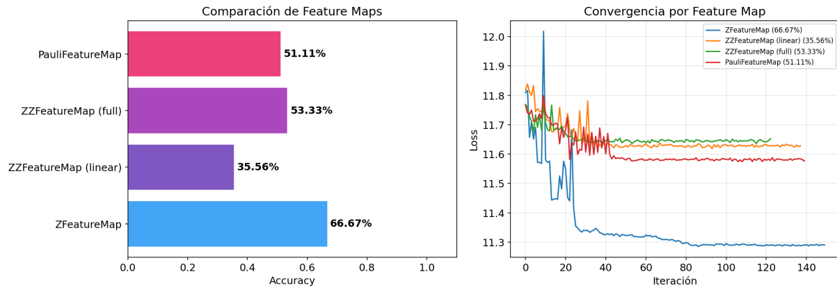
Figura 7: Izquierda: accuracy por feature map. Derecha: curvas de convergencia de la función de pérdida.
