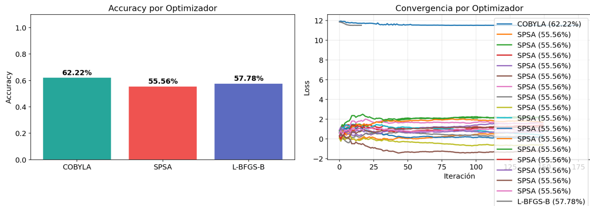
Figura 9: Izquierda: accuracy por optimizador. Derecha: curvas de convergencia de la función de pérdida.
