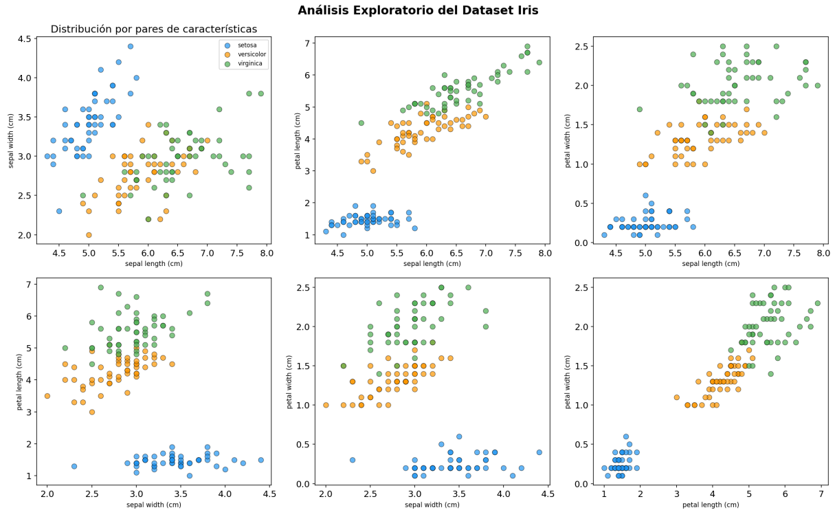
Figura 2: Distribución de las muestras de Iris por pares de características. Setosa (azul) es claramente separable de versicolor y virginica.
