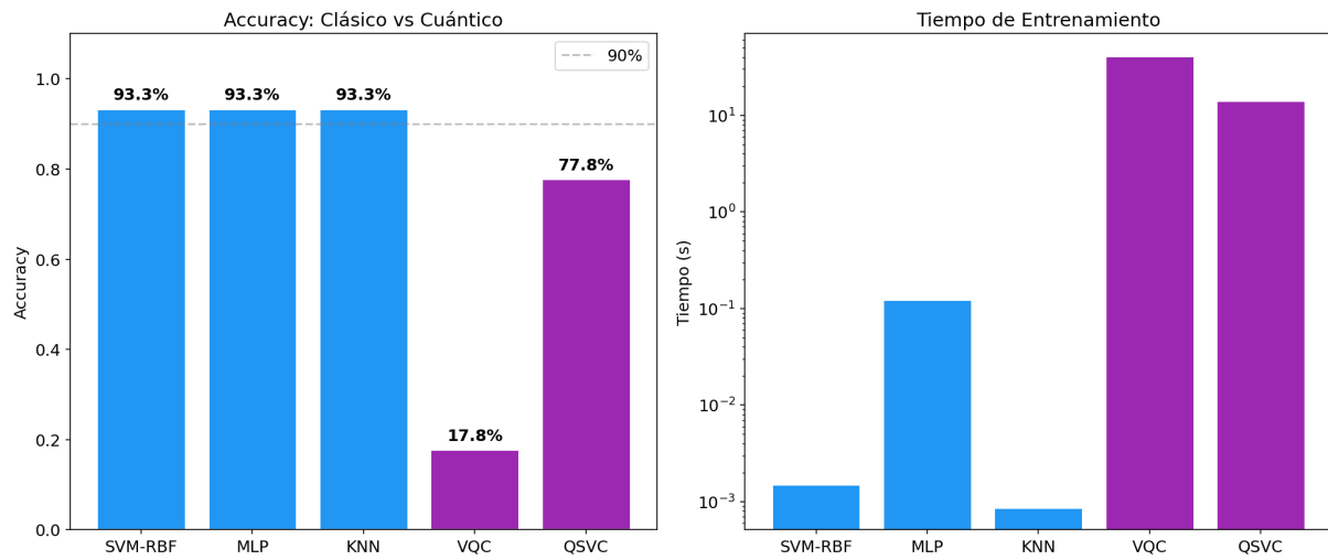
Figura 4: Izquierda: accuracy por modelo. Derecha: tiempo de entrenamiento (escala logarítmica). Azul = clásico, morado = cuántico.
