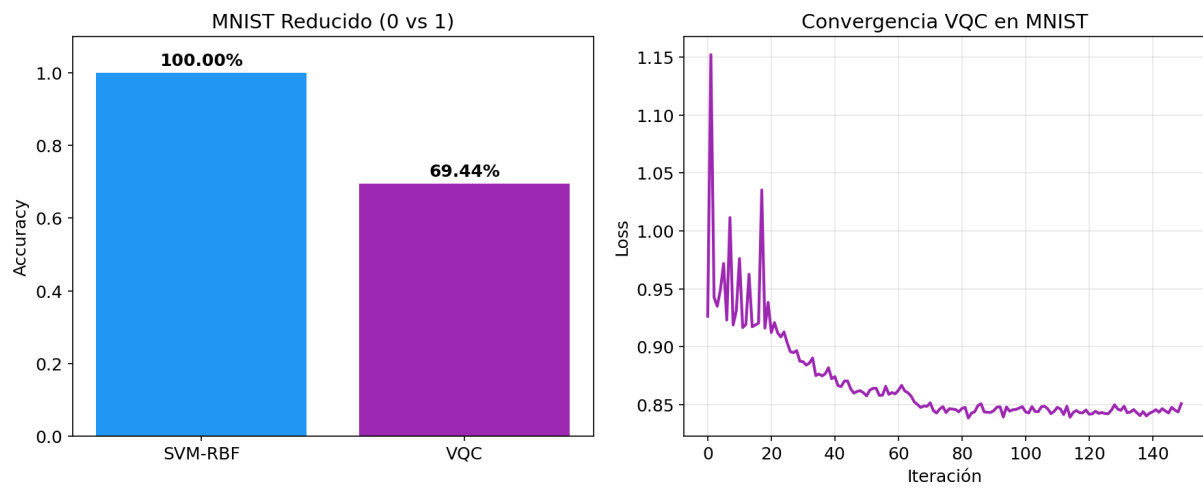
Figura 12: Izquierda: accuracy SVM vs VQC en MNIST reducido. Derecha: convergencia del VQC.
