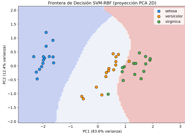
Figura 6: Frontera de decisión del SVM-RBF proyectada en las dos primeras componentes principales (PCA 2D).
