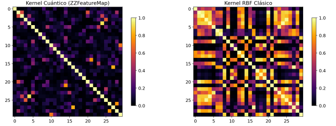
Figura 10: Izq: kernel cuántico (ZZFeatureMap). Der: kernel RBF clásico.
