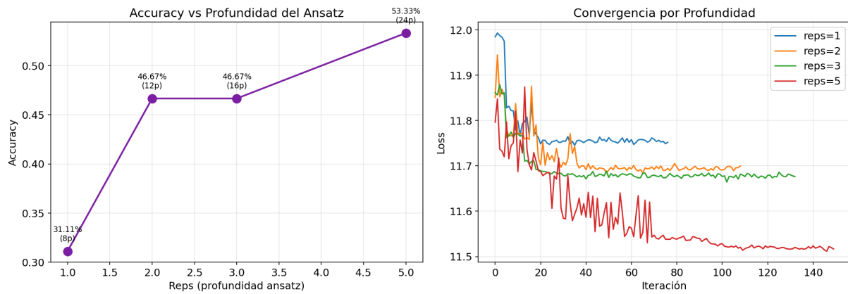
Figura 8: Izquierda: accuracy vs número de repeticiones del ansatz. Derecha: convergencia por profundidad.
